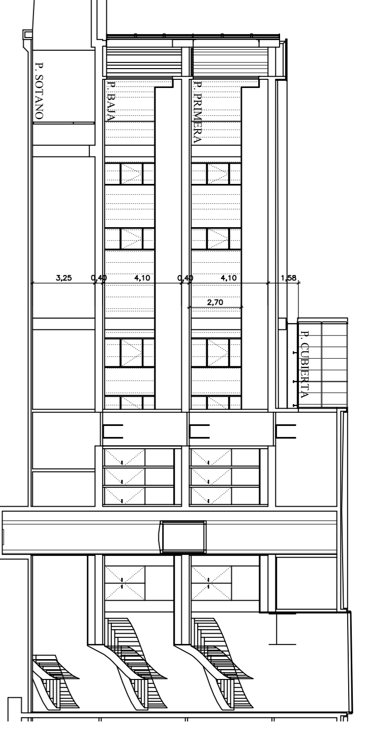
SECCION A-A'
